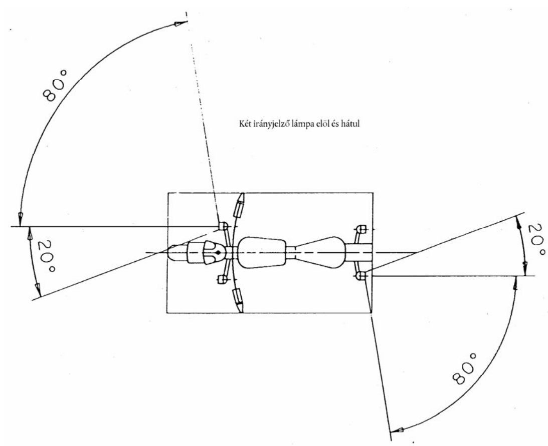
Elrendezési vázlat
