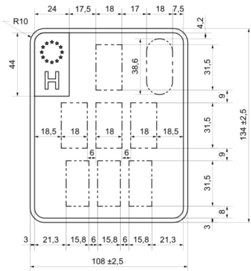
4. ábra: „E” típusú rendszámtábla rajzai
