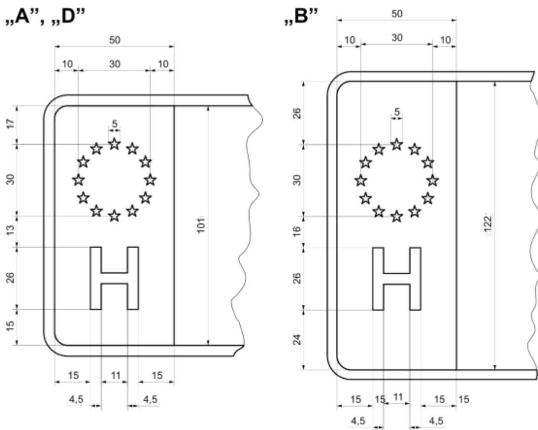
6. ábra: „A”, „D” és „B” típusú rendszámtáblák tagállamjelzésének méretei
