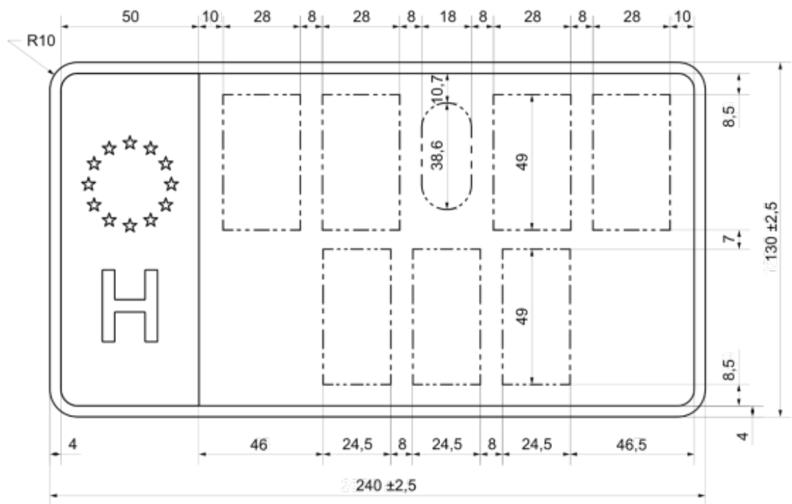
2. ábra: „B” típusú rendszám tábla rajzai
