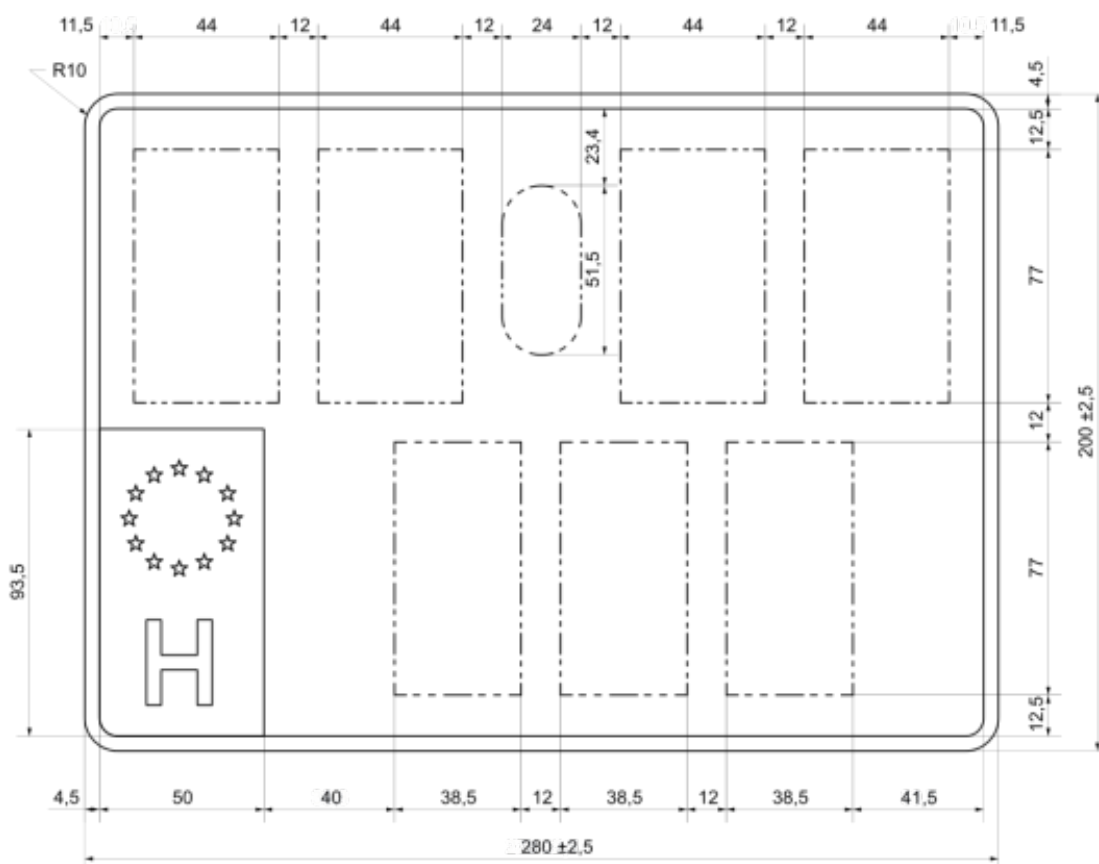
3. ábra: „C” típusú rendszám tábla rajzai
