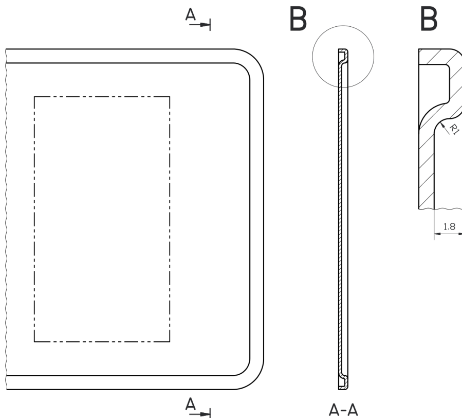
5. ábra: Rendszámtábla keretének és karaktereinek kialakítása
