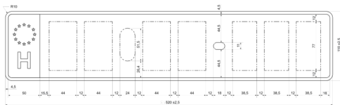
1. ábra: „A” és „D” típusú rendszámtáblák rajzai
