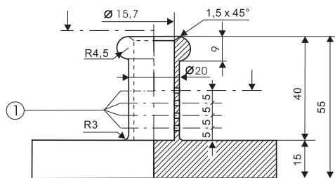
3. ábra: Talpas bronzhenger, egyik végén zárt: felülnézet és oldalnézet metszettel, mérték mm-ben
