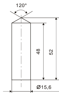
2. ábra: Hengeres bronzdugattyú, mérték mm-ben
