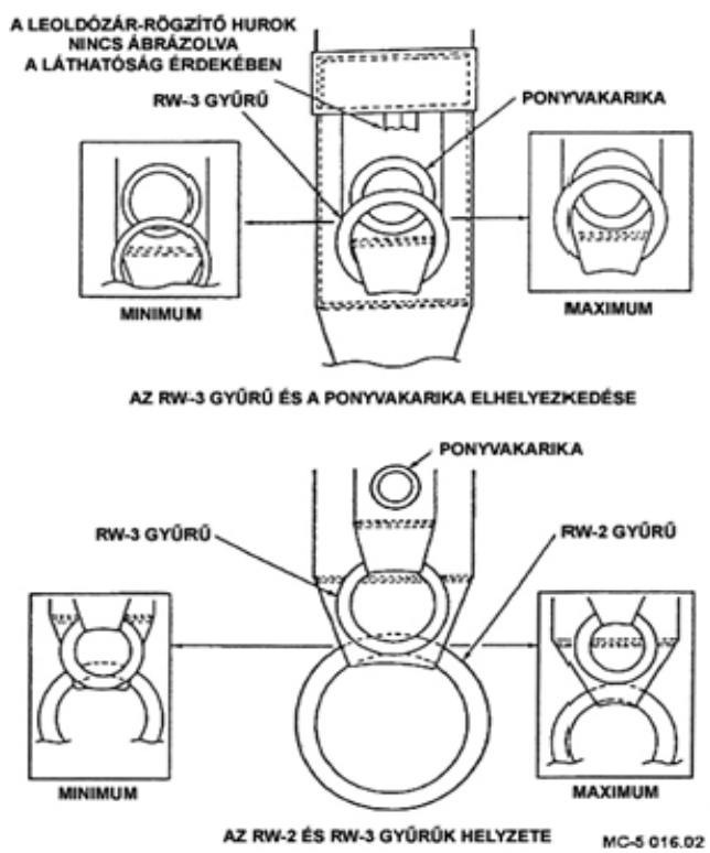
1. ábra A leoldózás megfelelő helyzete
