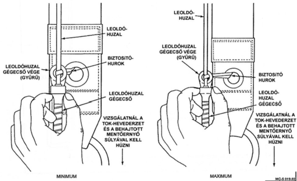
4. ábra Leoldózár-biztosító hurok helyzete
