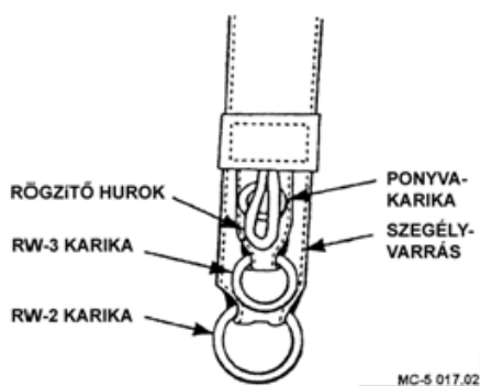
2. ábra RW típusú leoldózár felépítése
