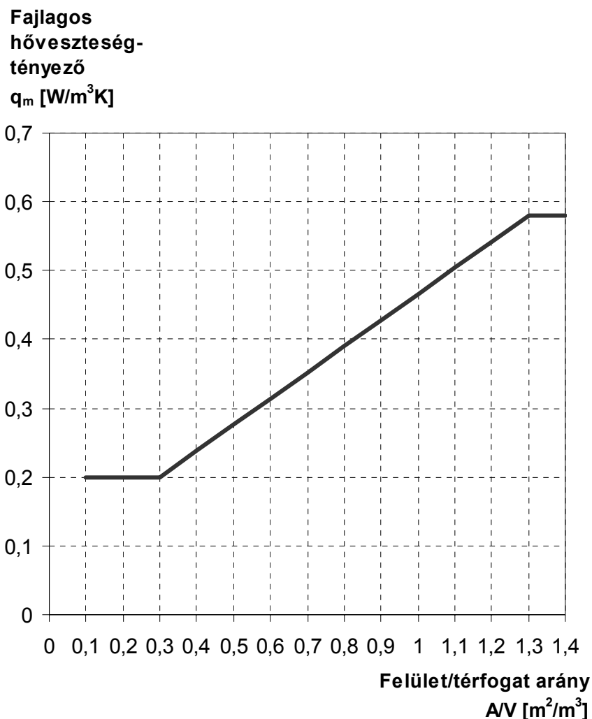
1. ábra: A fajlagos hővesztégtényező követelményértéke
